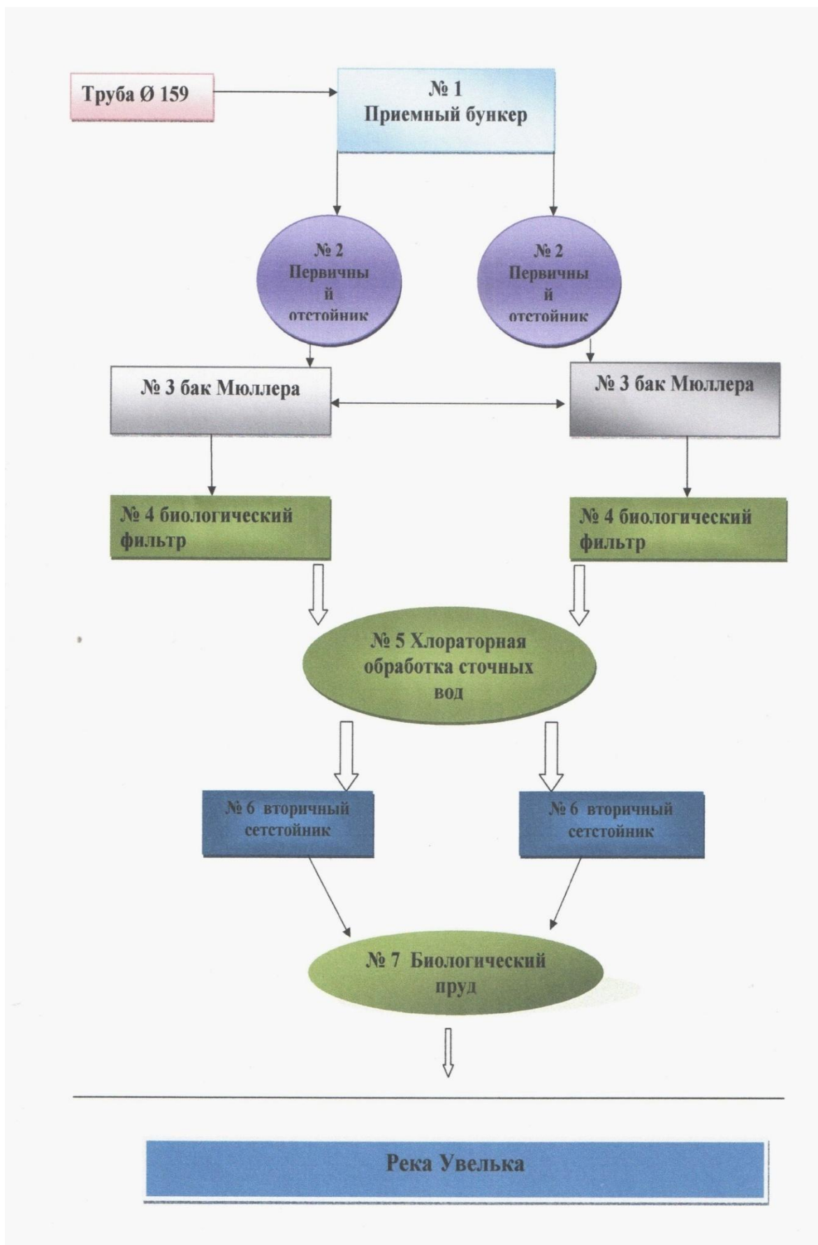
Рисунок № 9.1. Схема очистных сооружений с. Коелга
