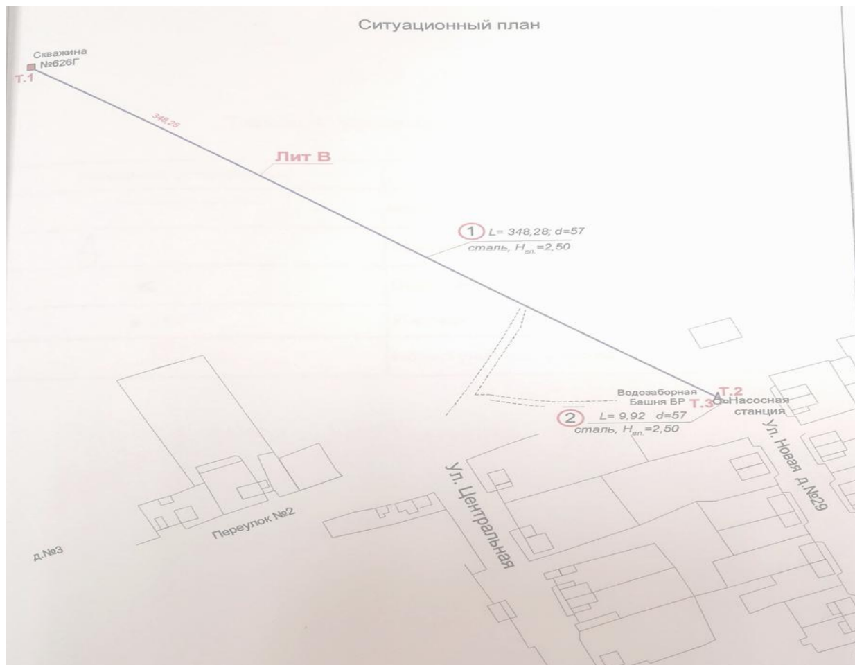
Рисунок 4.5. Схема ситуационного плана расположения скважин и водонапорных объектов водоснабжения в с. Долговка
