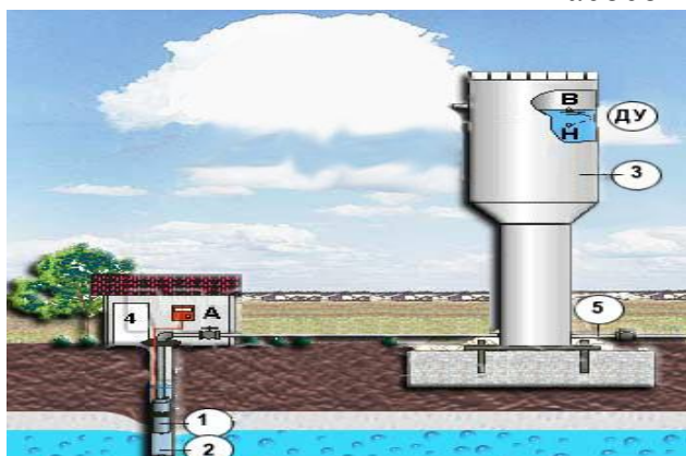
Рисунок № 1.1. Изображение водонапорной башни с погружным насосом.
