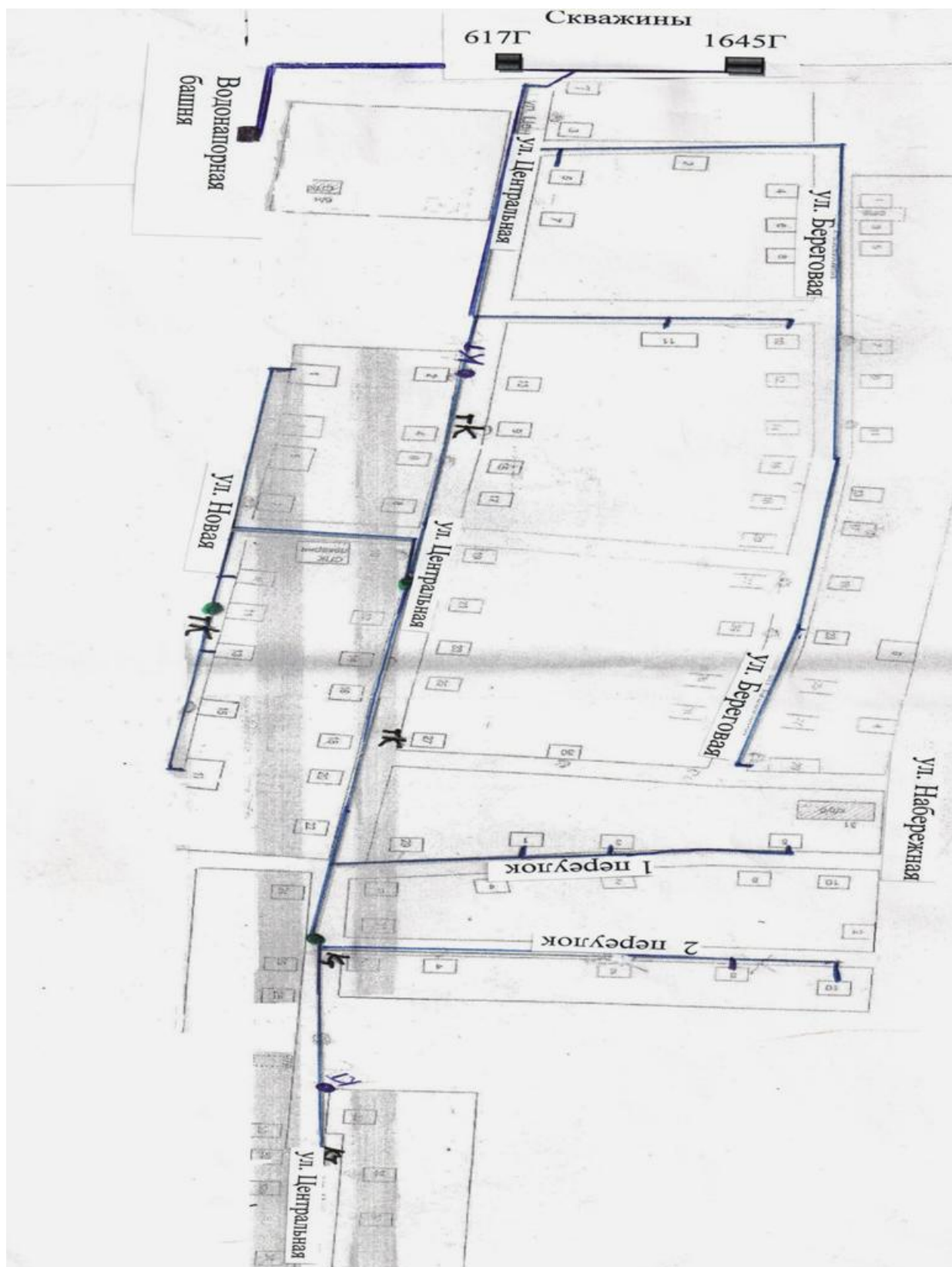
Рисунок 4.3. Схема сетей водоснабжения в д. Погорелка
